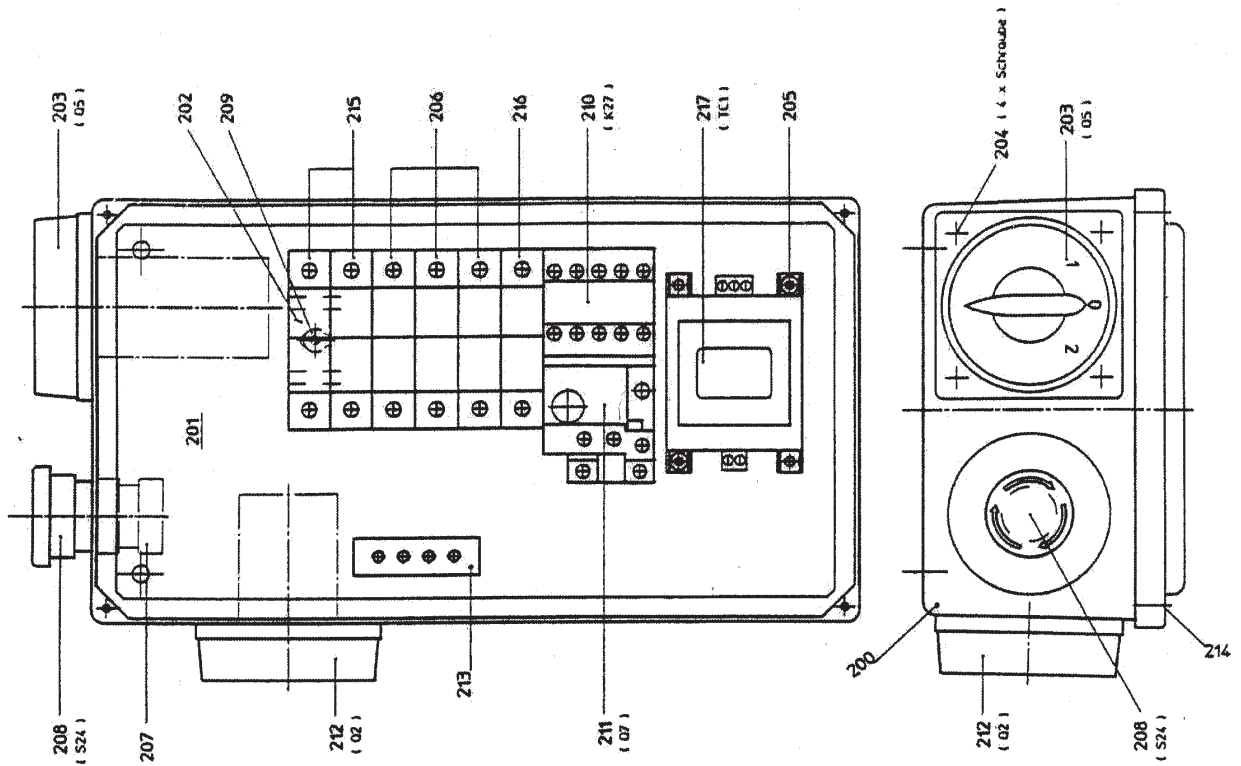
Cassetta impianto elettrico Electric box Boîte Eléctrique Schaltkasten Caja Eléctrica
